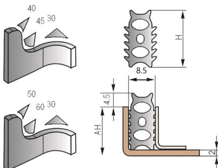
黑色发泡EPDM唇型密封胶条，肖氏硬度25°
